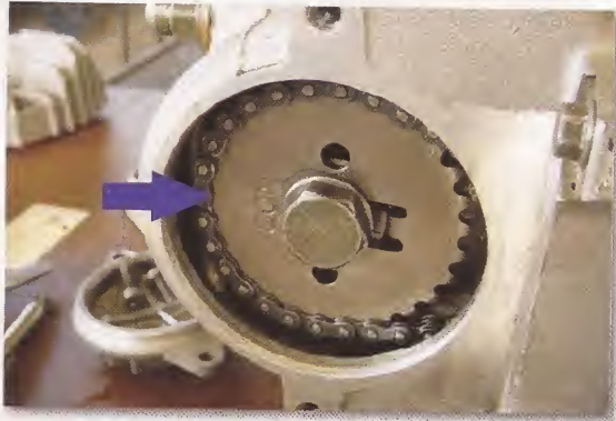
Toma de tiempo mecánico en motor horizontal
